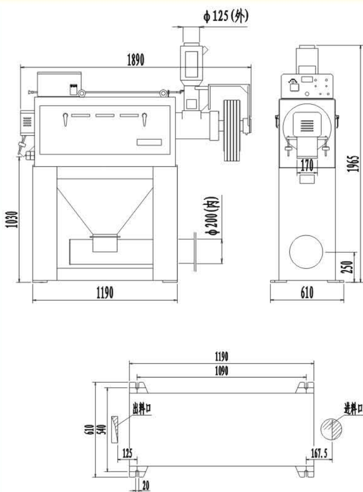
(外形尺寸与地脚安装图)
